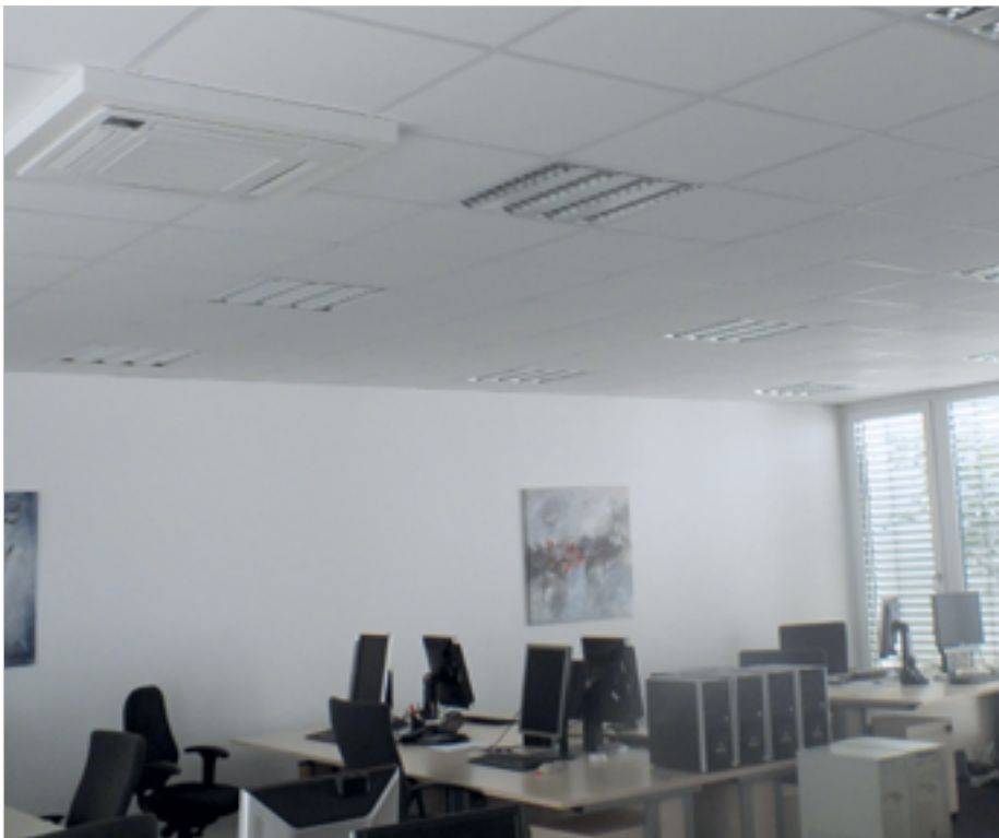
Ein Großraumbüro klimatisiert mit VRF 4 Wege Kassetten
